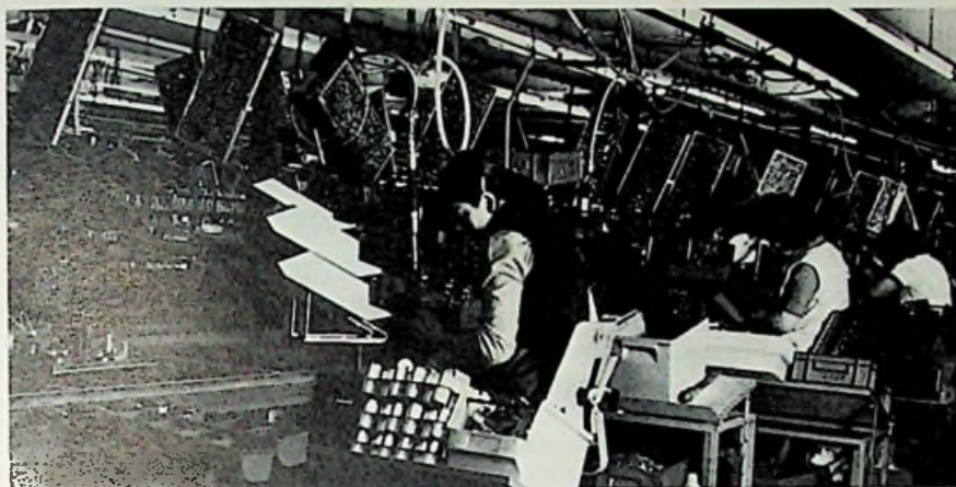
Montageband nach der Arbeitsstrukturgestaltung
