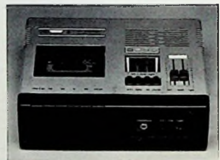
Marke: Teleton Modellname: CD 200 Erstlieferung a. d. Handel: Nov. 75 Endverkaufspreis: bei etwa 600 DM Bandart-Umschaltung: von Hand Rauschunterdrückung: Dolby
