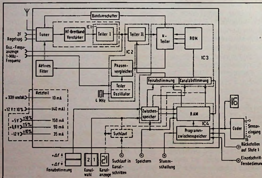
Die PLL-Schaltung mit 16 Programm-Speicherstellen
