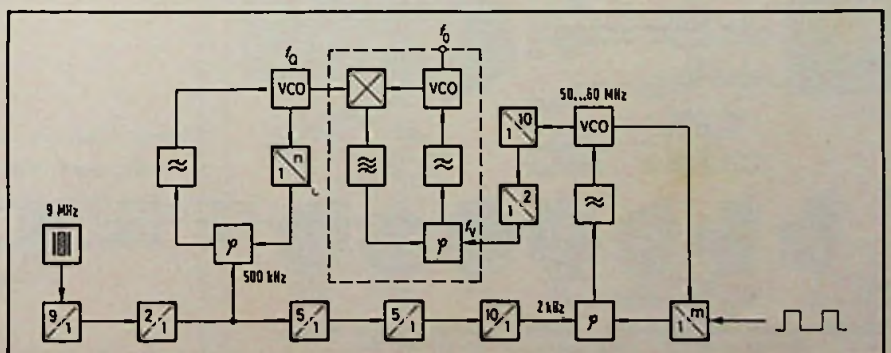
Bild 2. Erweiterung der Anordnung nach Bild 1 zu einer quasikontinuierlichen Veränderung der Frequenz „
