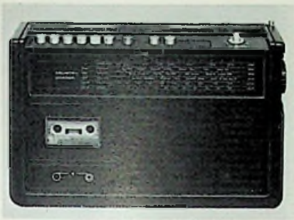
Marke: Graetz Modellname: Travel Corder 307 Erstlieferung a. d. Handel: Okt. 75 Endverkaufspreis: bei etwa 370 DM Bereiche: UKW, KW, MW, LW Batteriebestückung: 5 Monozellen Gewicht mit Batterien: 3,6 kg
