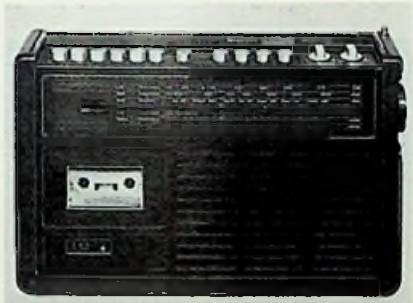
Marke: Graetz Modellname: Country Corder 307 Erstlieferung a. d. Handel: Okt. 75 Endverkaufspreis: bei etwa 280 DM Bereiche: UKW, MW Batteriebestückung: 5 Monozellen Gewicht mit Batterien: 3,4 kg
