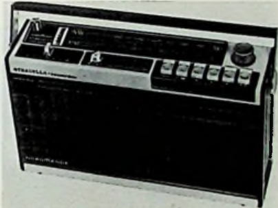
Marke: Nordmende Modellname: stradella + recorder Erstlieferung a. d. Handel: Nov. 75 Endverkaufspreis: bei etwa 300 DM Bereiche: UKW, MW, LW Batteriebestückung: 4 Monozellen Gewicht mit Batterien: 3 kg
