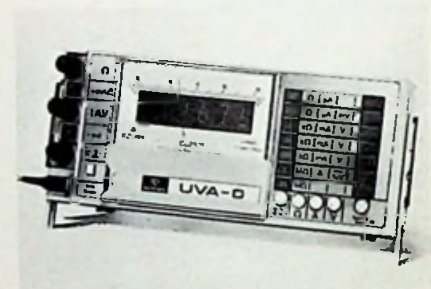
Hersteller: Norma Meßtechnik Bezeichnung: UVA-D Anzeige: Röhren, \pm 1999 Bereiche: 29 (DCV, DCI, ACV, ACI, R) Auflösung: 0,1 mV; 10 m \Omega Meßfehler: \pm 0,1\% ; \pm 0,8\% Stromversorgung: Netz Gewicht: 1,7 kg Preis: 1145 DM
