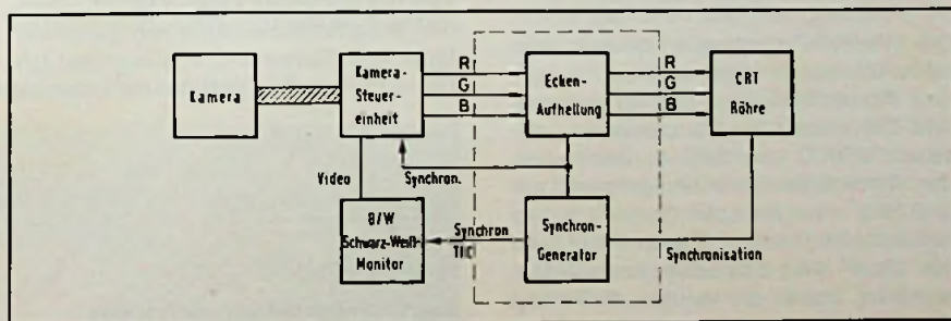
Das Block-Diagramm des hochauflösenden Systems
